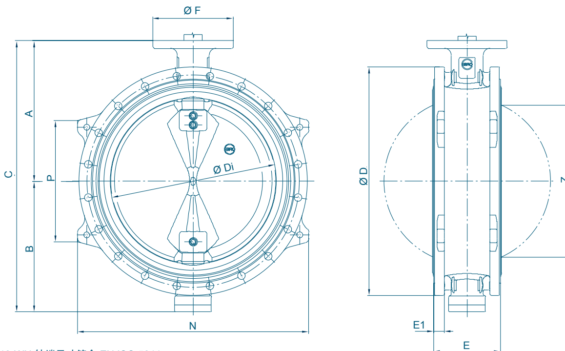
F012-WN 轴端尺寸符合 EN ISO 5211
